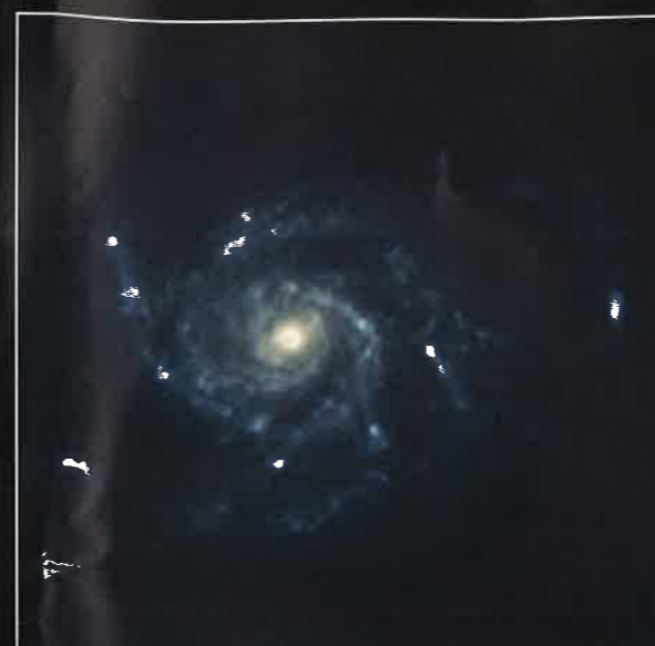
Zgoraj: Spiralna galaksija M 101, imenovana Vetrnica, v ozvezdju Velikega medveda. Desno: Planetarna meglica Ročka (M 27) v ozvezdju Lisičke. Spodaj: Dvojna kopica v Perzeju.
